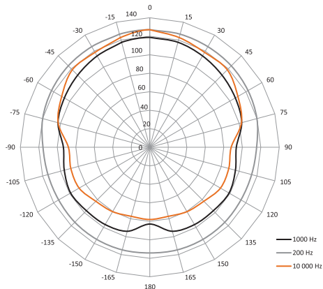
SAM-15 - 标准的水平覆盖范围
