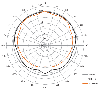
SAM-8 - 标准的水平覆盖范围
