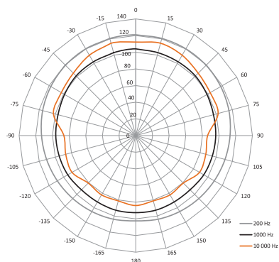
SAM-5 - 标准的水平覆盖范围
