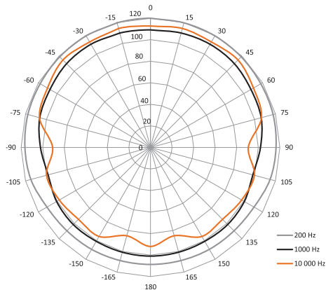
SAM-15 - 标准的垂直覆盖范围
