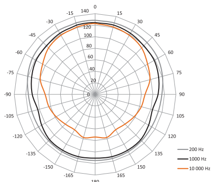
SAM-12 - 标准的水平覆盖范围
