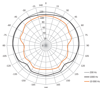
SAM-12 - 标准的垂直覆盖范围
