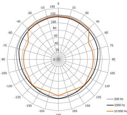
SAM-8 - 标准的垂直覆盖范围
