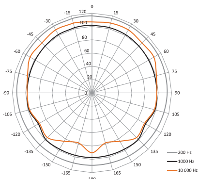
SAM-5 - 标准的垂直覆盖范围
