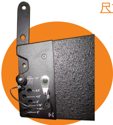
角阶调节系统
